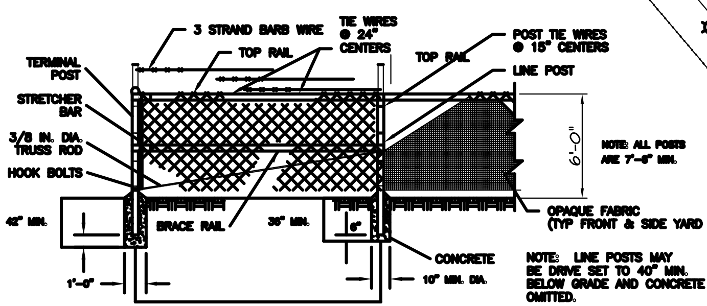
2 FENCE DETAIL SDI N.T.S.
